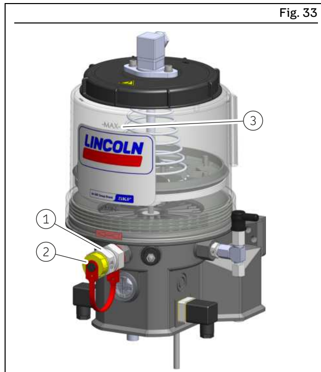
Filling via the optional fill connection
